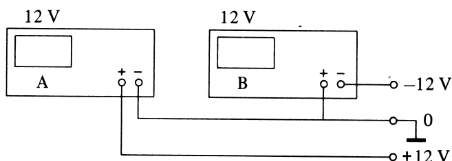
Fig. 10. Bipolar spændingsforsyning.
