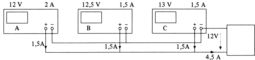
Fig. 7. Parallelforbindelse af tre SN17-enheder
